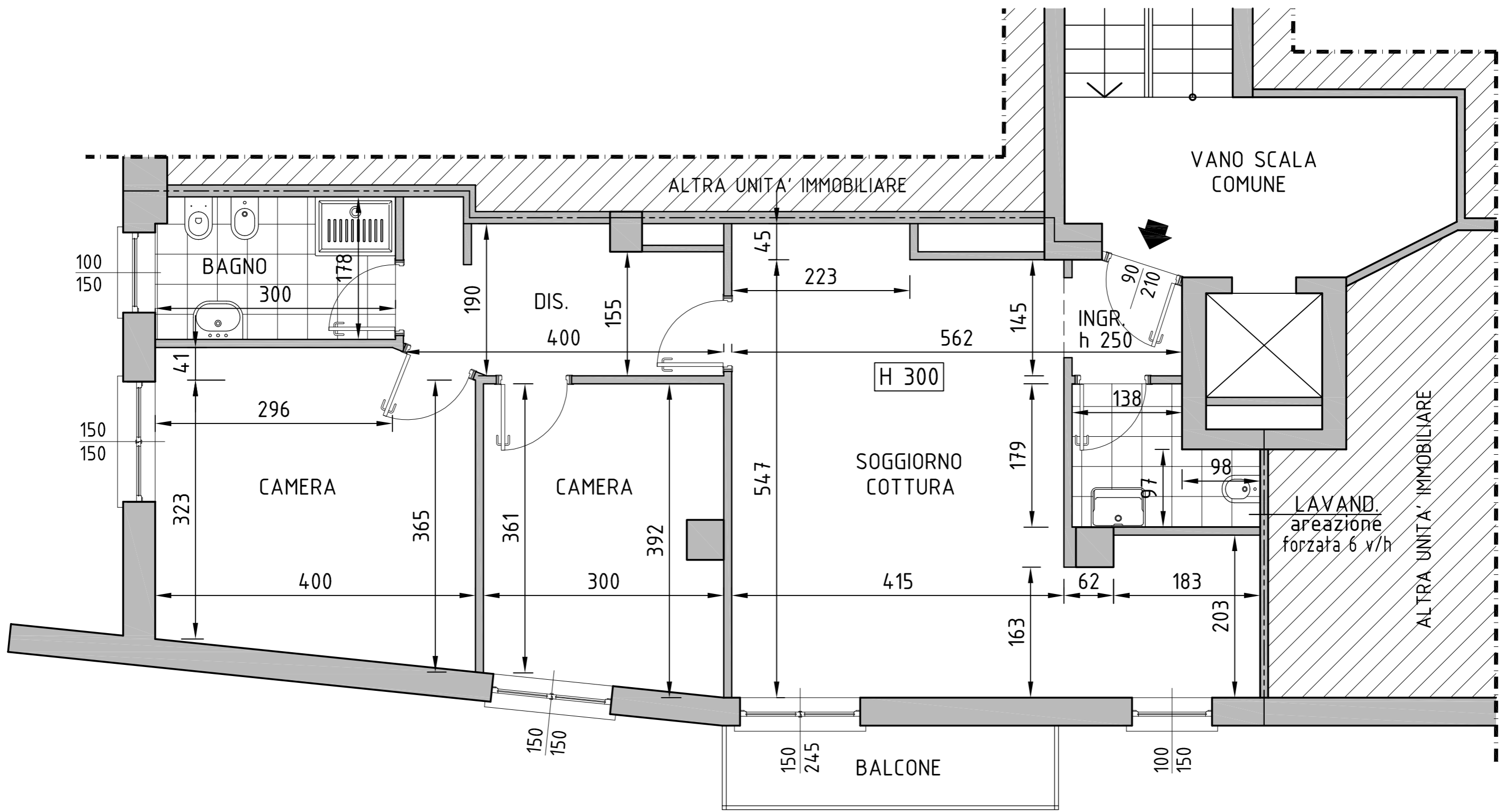
PLANIMETRIA PIANO SECONDO - Stato di Progetto
